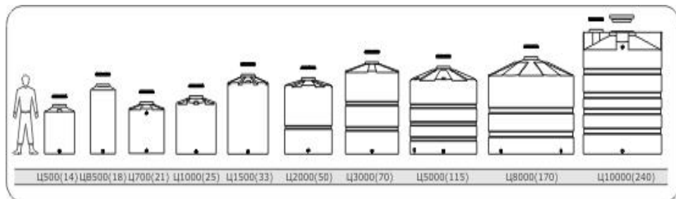
Рис.1 Виды цилиндрических емкостей
