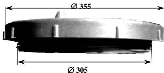
Рис.1.1 Вид крышки Д
