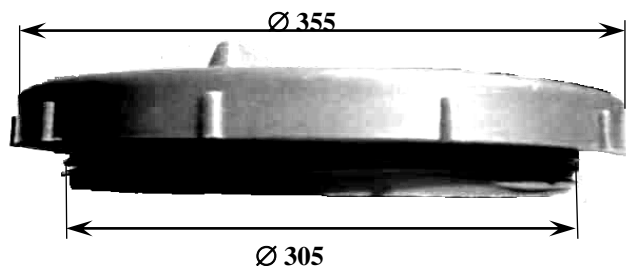
Рис.1.1 Вид крышки Д
